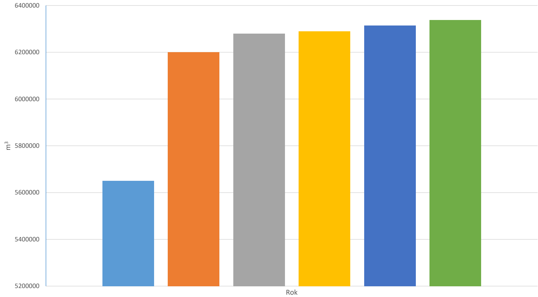
Dynamika zmian zapasu miąższości w latach 2005-2021
